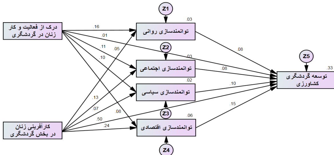
شکل ۲ - تحلیل مسیر مدل پژوهش
